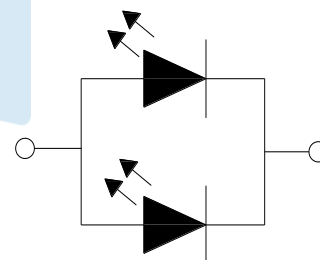
Fig.1-4 Polarity 极性
